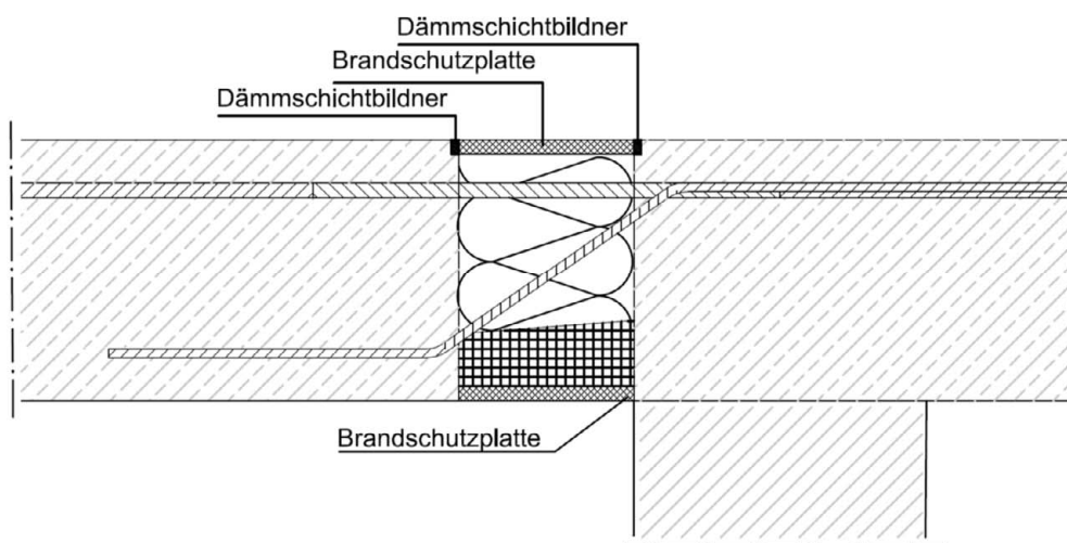
Abb. 1: prinzipielle Ausführung mit freiliegender Fuge
