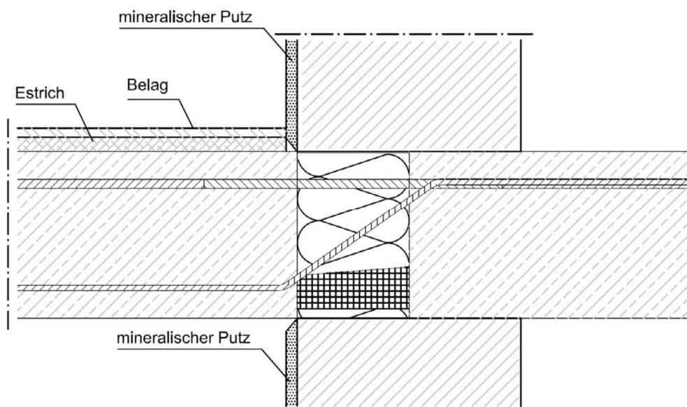
Abb. 2: prinzipielle Ausführung mit eingeschlossener Fuge
