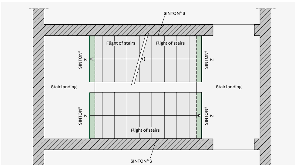
Anordnungsvorschlag SINTON® Z – Grundriss
