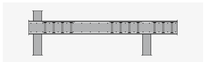
Bild 5: JORDAHL® Durchstanzbewehrung JDA mit Doppelkopfkankern
