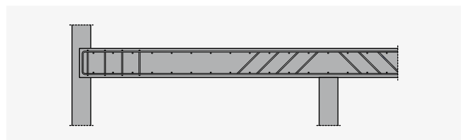
Bild 4: Flachdecke mit Bügeln und Schrägaufbiegung
