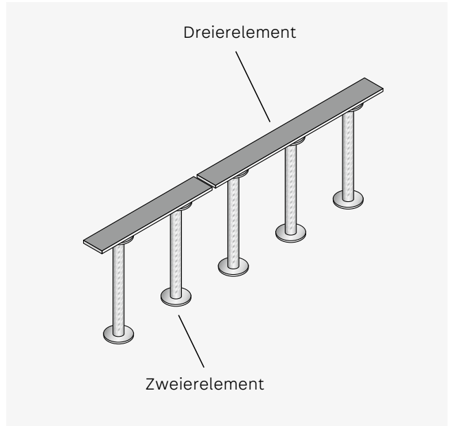
JDA-Standardelemente (geteilt)
