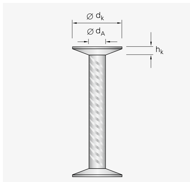
Doppelkopfanke gerippt
