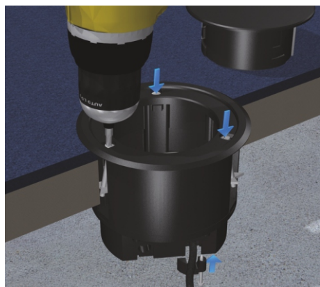
4 | Montaż zacisku kablowego Zamontować od dołu jednostki docisk kablowy odciążający oprzewodowanie i zabezpieczyć kable. Dokręcić trzy łapki montażowe jednostki za pomocą śrub krzyżakowych.
