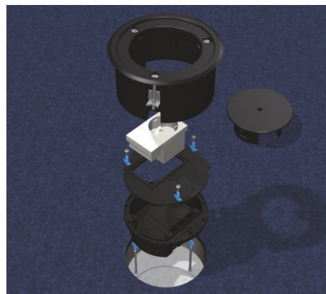
3 | Montaż gniazda W celu podłączenia gniazda należy rozmontować kasetę, wprowadzić kabel i podłączyć go do gniazda. Następnie zamontować maskownicę z gniazdem w puszcze instalacyjnej.
