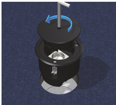
2 | Pokrywa wyprowadzenia kablowego Przy użyciu klucza torx (należy zamówić osobno), otworzyć pokrywę jednostki, obracając klucz w kierunku przeciwnym do ruchu wskazówek zegara.
