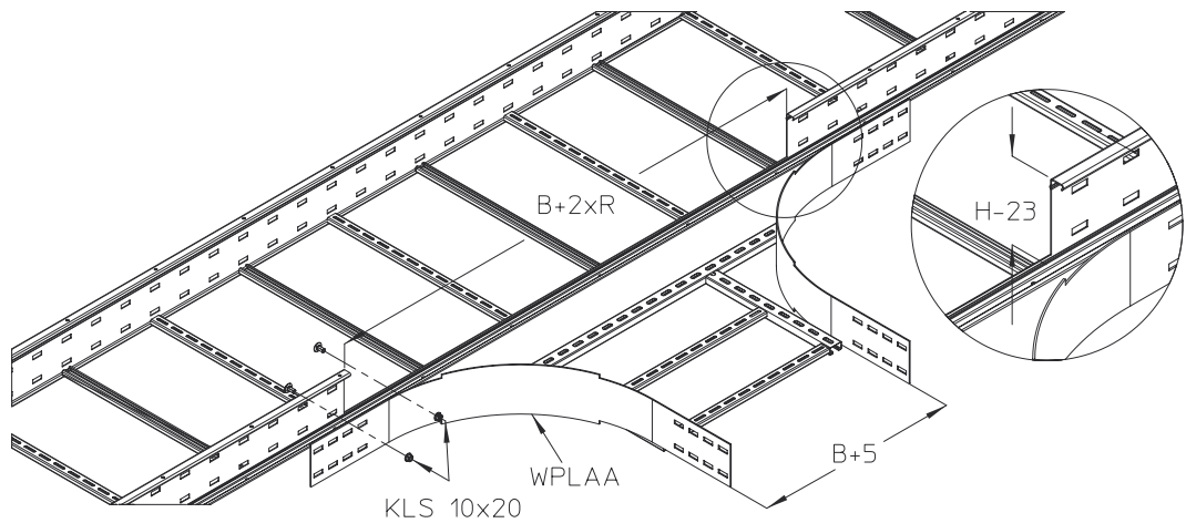
Wykonanie trójnika - odgałęzienia bocznego
