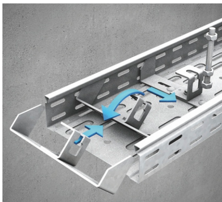
8 | Zawiesie centralne dla tras kablowych o szerokości do 300 mm
