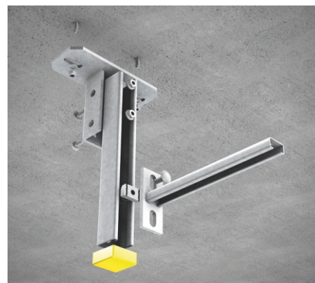
14 | Montaż sufitowy płyty czołowej BGA 41 z kształtownikiem KHA 41
