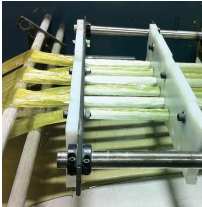
Herstellung von FIBERNOX® V-ROD im Pultrusionsverfahren
