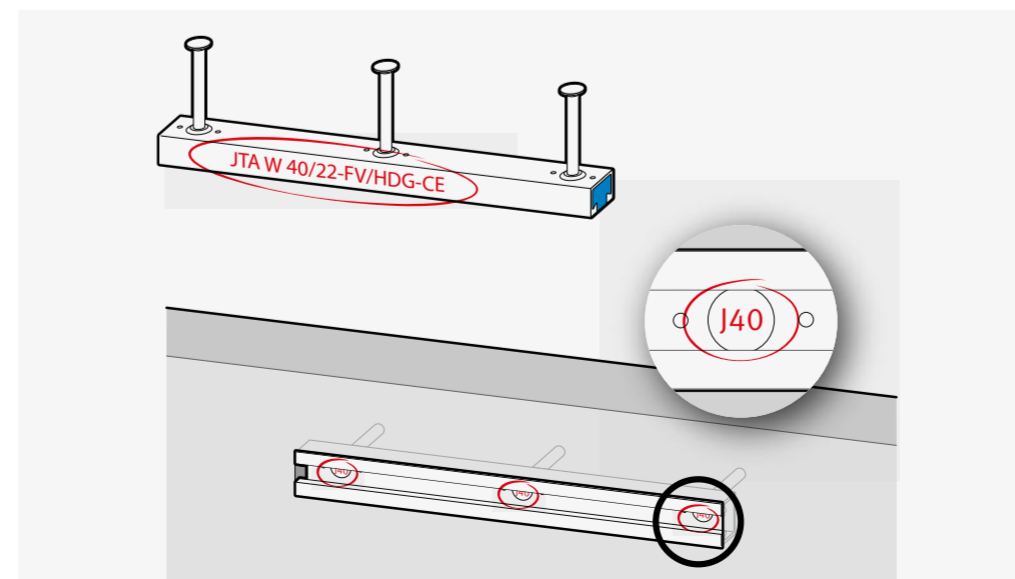
Beispiel Darstellung Ankerschiene Example of anchor channel
