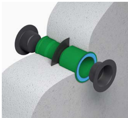
Transwand mit Muffe und Überziehmuffe
