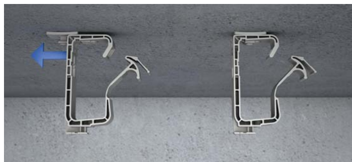
Montage unter Verwendung des Befestigungssockels (BFS K)
